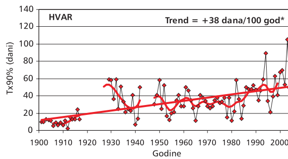
Slika 5-3: Lijevo: broj dana s minimalnim (Tn 90%); desno: broj dana s maksimalnim (Tx 90%) temperaturama zraka višim od 90-og percentila i trendovi za razdoblje 1901. – 2004. (* signifikantno na razini \alpha=0,05 )
