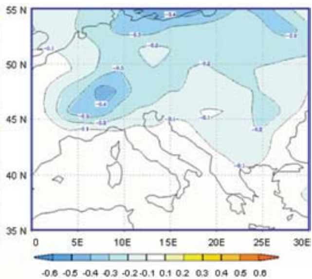
Slika 5-6: Sezonski srednjak za snježnu oborinu u sadašnjoj klimi (1980. – 1990.), lijevo i razlika između buduće (2040. – 2050.) i sadašnje klime (desno). Izolinije svakih 0,2 mm/dan (lijevo); 0,1 mm/dan (desno)
