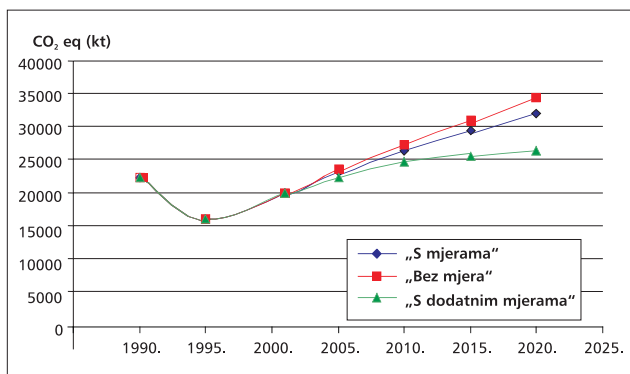
Slika 4-2: Projekcije emisije stakleničkih plinova za sektor Energetika
