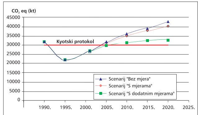
Slika 4-1: Projekcije emisije stakleničkih plinova u Republici Hrvatskoj za razdoblje 1990. – 2020. godine
