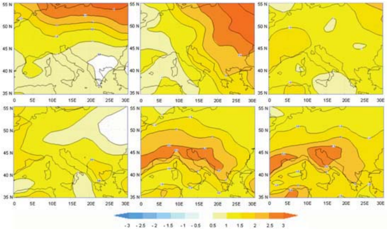
Slika 5-4: Sezonski srednjaci razlika u temperaturi na 2 m između buduće (2040. – 2050.) i sadašnje (1980. – 1990.) klime, za zimu (gornji niz slika) i ljeto (donji niz slika) za tri realizacije EH5OM modela. Izolinije svakih 0,5 stupnjeva
