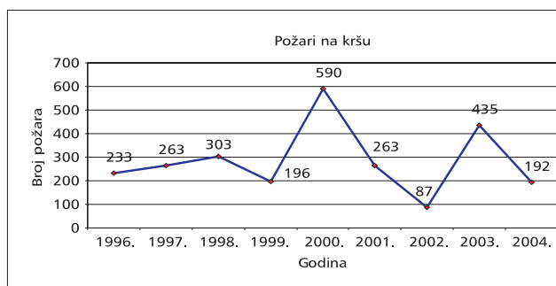
Slika 5-11: Broj požara (lijevo) i temperaturni prosjeci za razdoblje lipanj-kolovoz (desno), u krškom području Hrvatske u razdoblju 1996. – 2004. godine
