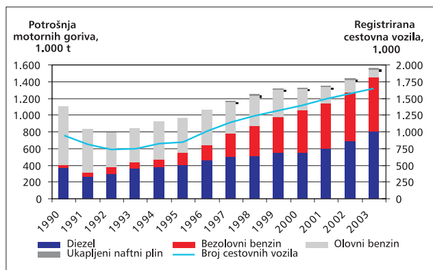
Slika 1-7: Broj vozila i potrošnja goriva u cestovnom prometu (1990. – 2003.)
