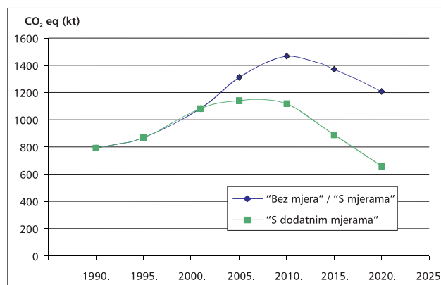
Slika 4-5: Projekcije emisije stakleničkih plinova za sektor Otpad
