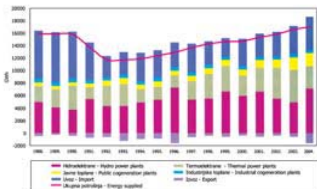
Slika 1-4: Bilanca električne energije u Hrvatskoj od 1988. do 2004. godine
